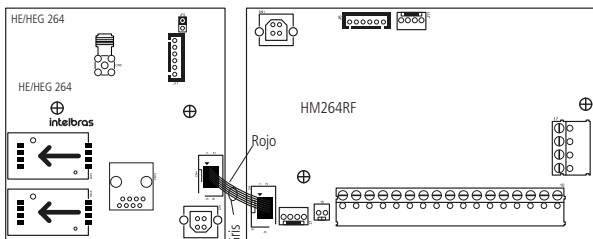
Esquema de conexión módulos de comunicación
